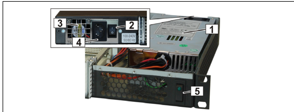
Figure 2: Netzgerät (Dargestellt am 1 HE System)
