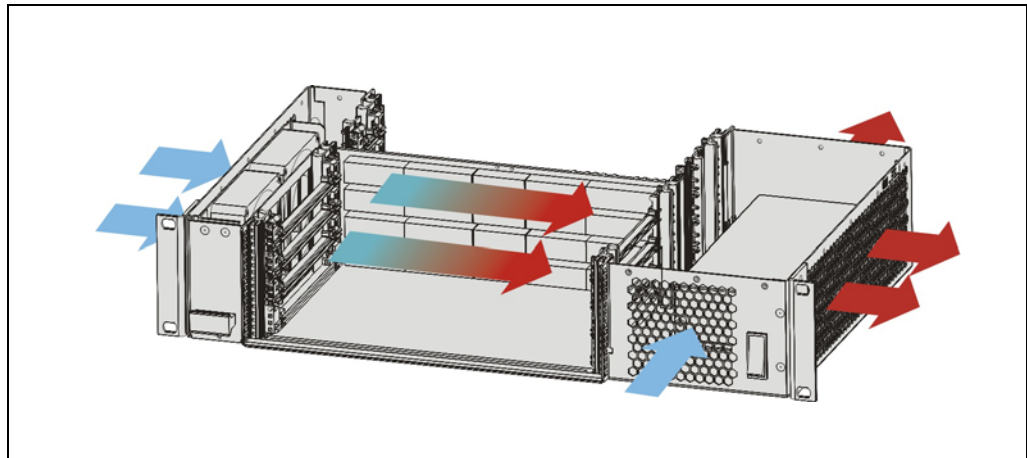
Figure 5: Entwärmung
